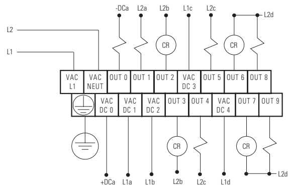
Output Wiring
