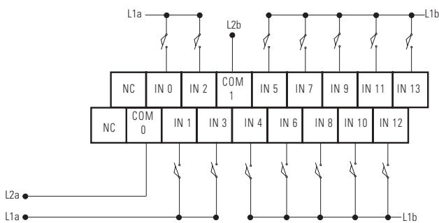
Input Wiring
