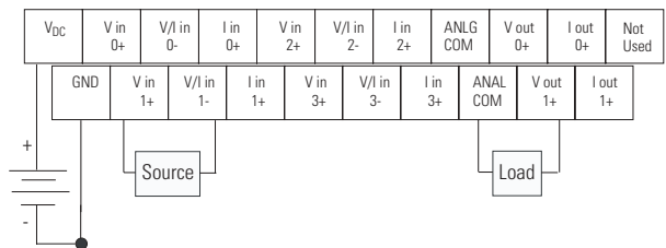
1791D-N4CV2X – Voltage
