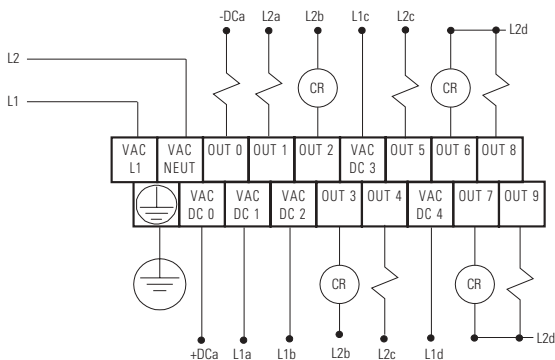
Output Wiring
